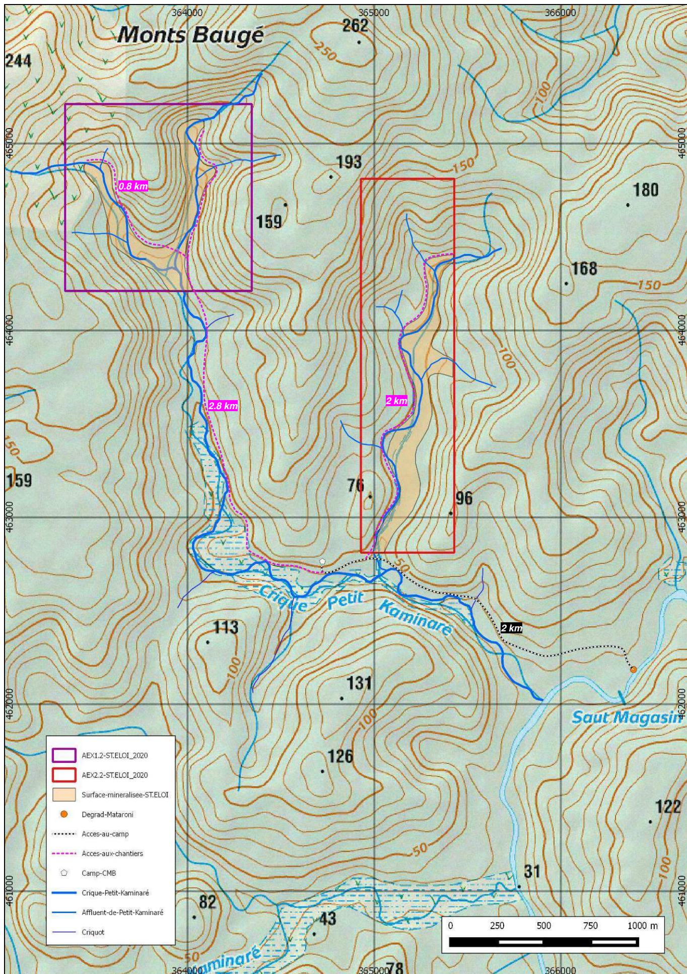
Plan de projet dans le cadre des AEX « crique Petit Caminaré » de la SARL SAINT-ELOI d'après la carte IGN au 1/17 500° en RGFG95 UTM22
