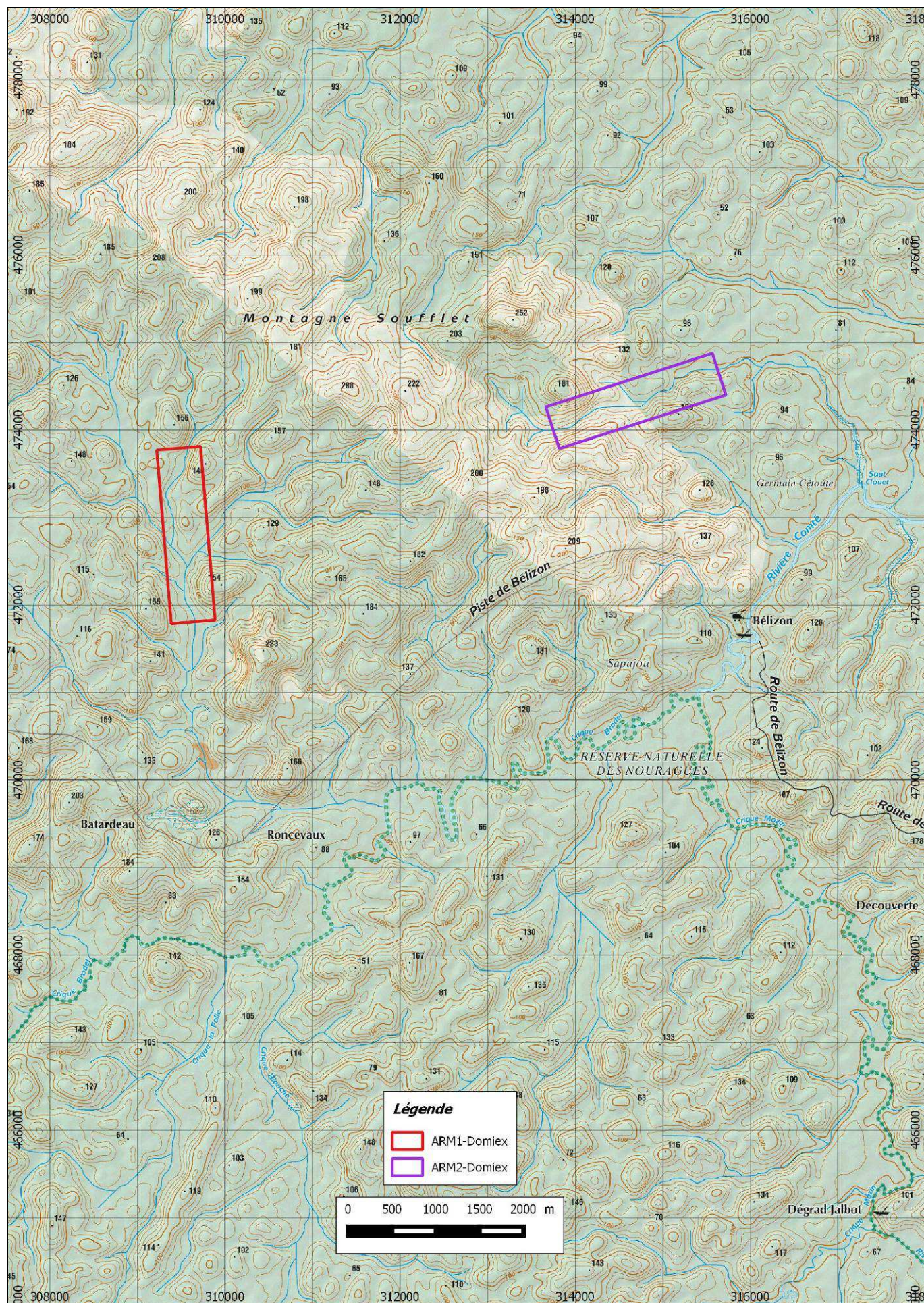
Carte de situation de l'ARM Belizon (zone Soufflet-Clouet), SARL DOMIEX, d'après la carte IGN au 1/50 000° en RGFG95 UTM22
