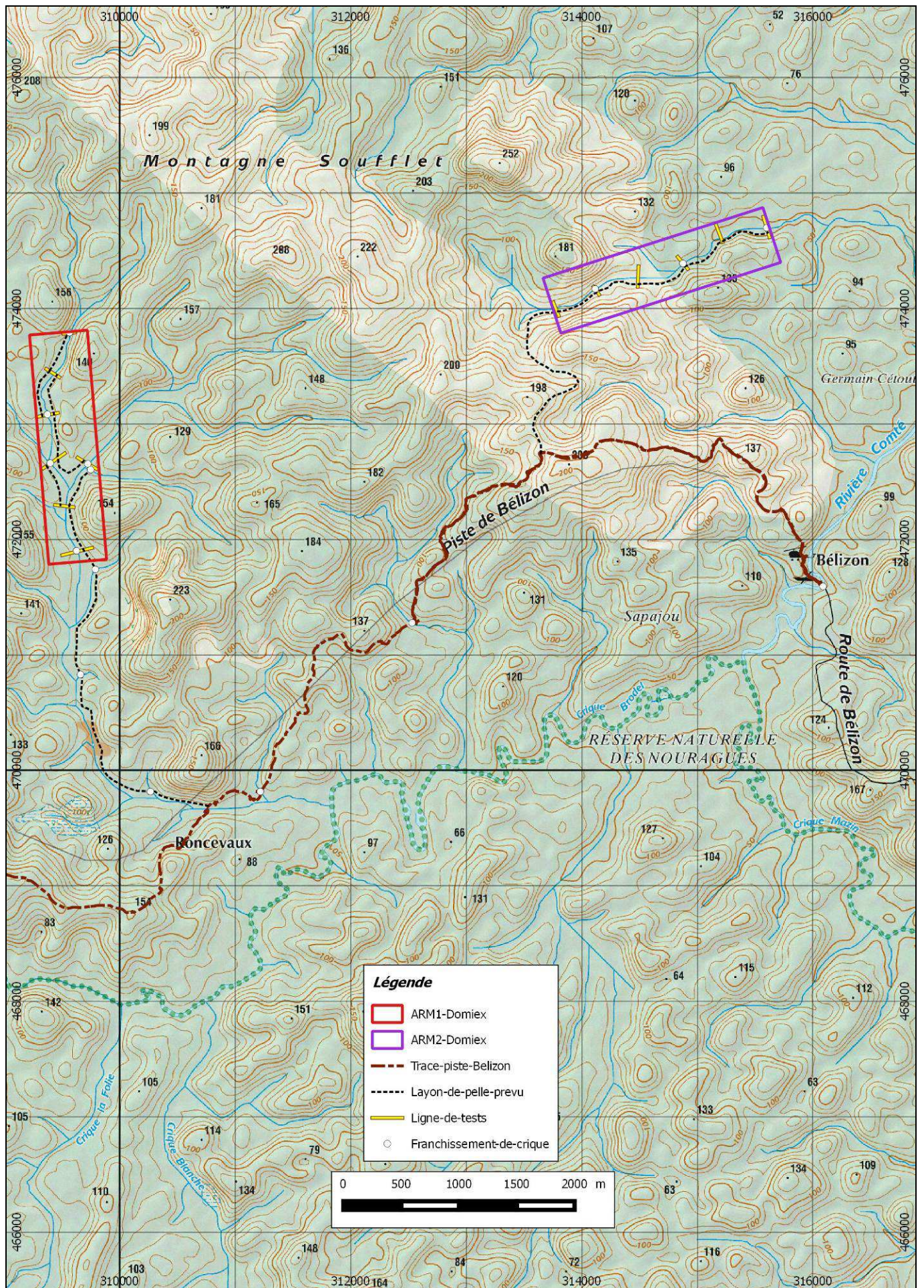
Schéma de pénétration du domaine forestier dans le cadre de l'ARM Belizon (zone Soufflet-Clouet), SARL DOMIEX, d'après la carte IGN au 1/50 000° en RGFG95 UTM22
