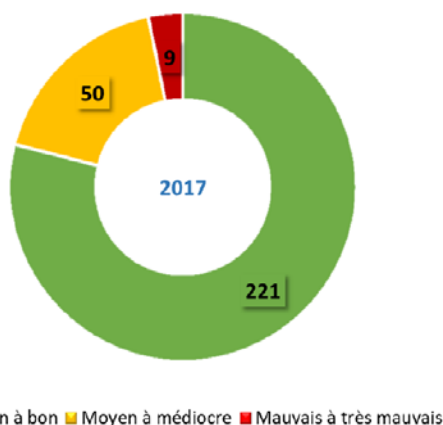
Figure 8 : Bilan des indices de qualité de l'air (IQA) à la station Brady en nombre de jour [DR23]
