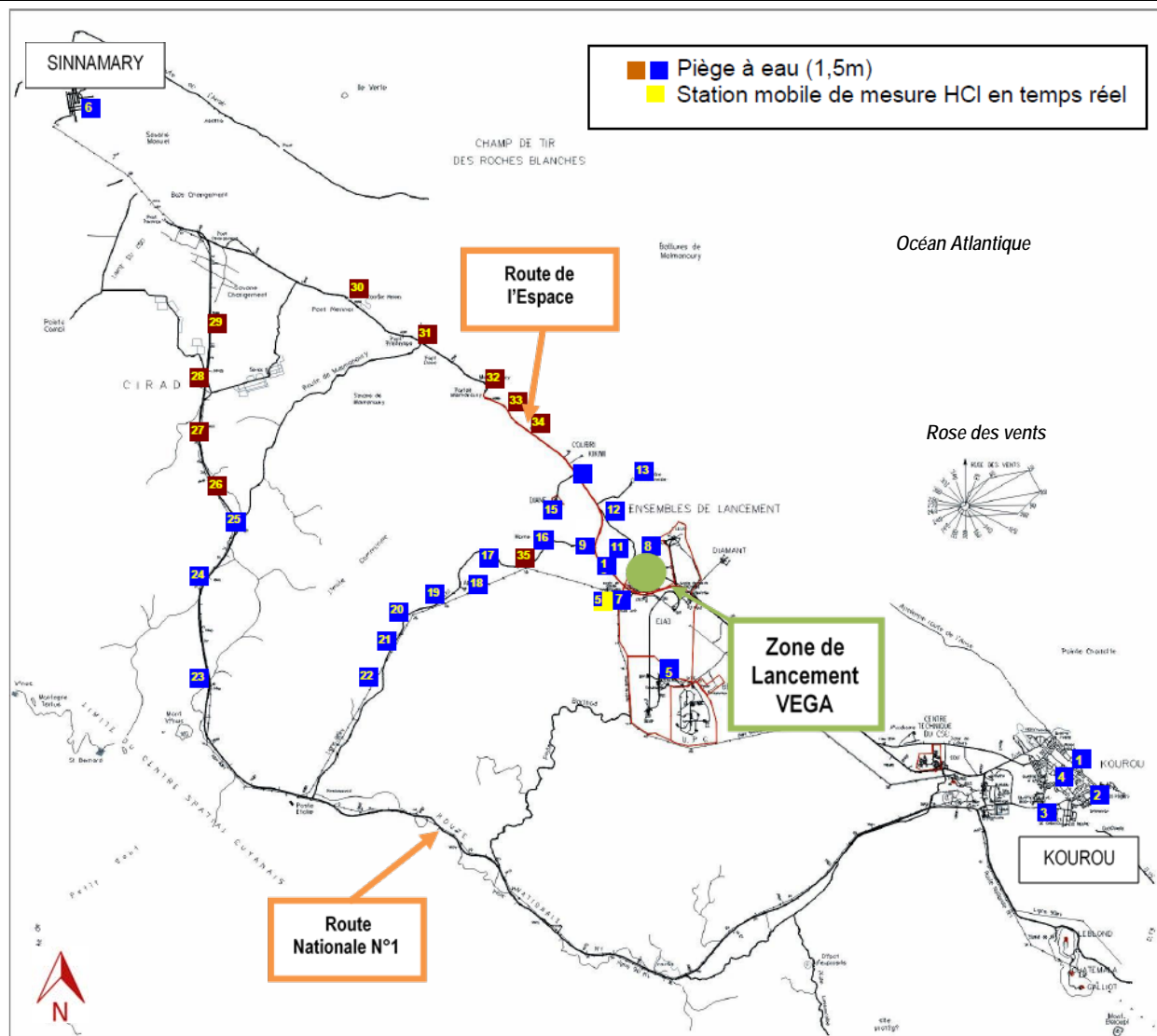
Figure 6 : Cartographie d'implantation des capteurs en champ lointain
