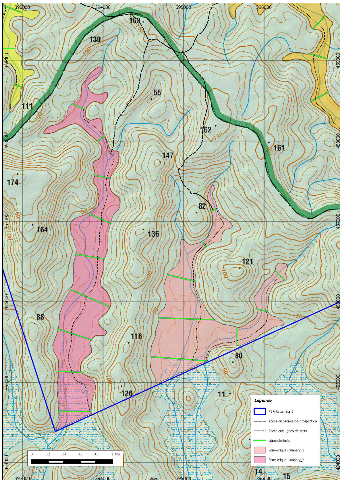
ANNEXE 4e : Plan de projet SANDS RESSOURCES - DOTM Puits de reconnaissance sur les zones n°6 et 7 (criques Ouany Est et Ouest) PER n°33-2019 d'après la carte IGN au 1/20 000° en UTM22, RGFG95
