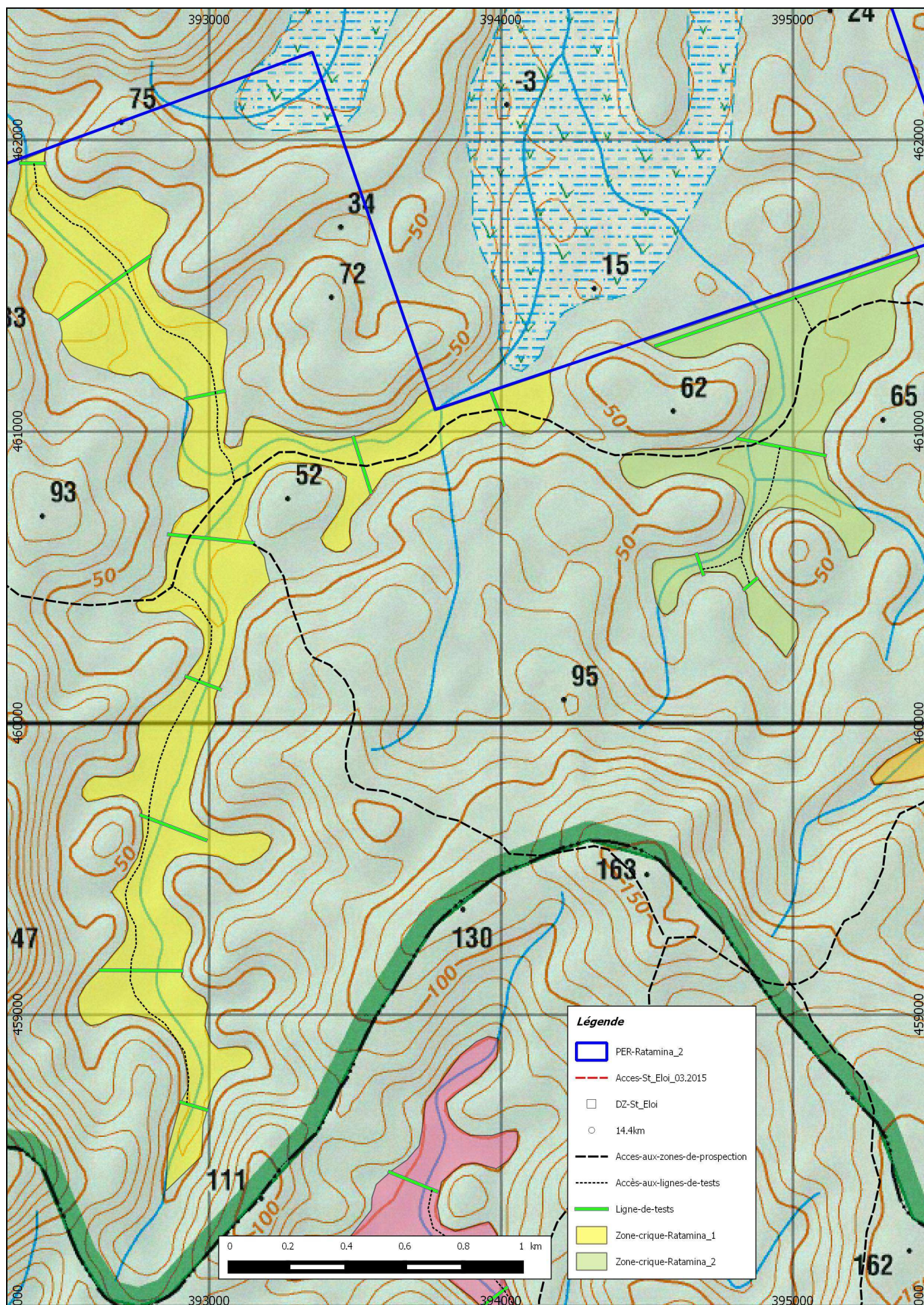
ANNEXE 4c : Plan de projet SANDS RESSOURCES - DOTM Puits de reconnaissance sur les zones n°2 et 3 (criques Ratamina Ouest et Est) PER n°33-2019 d'après la carte IGN au 1/15 000° en UTM22, RGFG95
