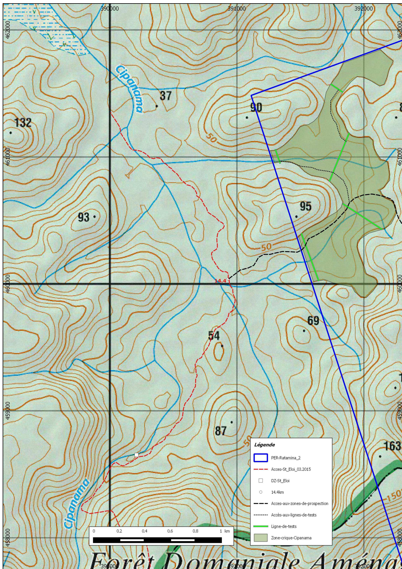
ANNEXE 4b : Plan de projet SANDS RESSOURCES - DOTM Puits de reconnaissance sur la zone n°1 (crique Cípanama) PER n°33-2019 d'après la carte IGN au 1/15 000° en UTM22, RGFG95
