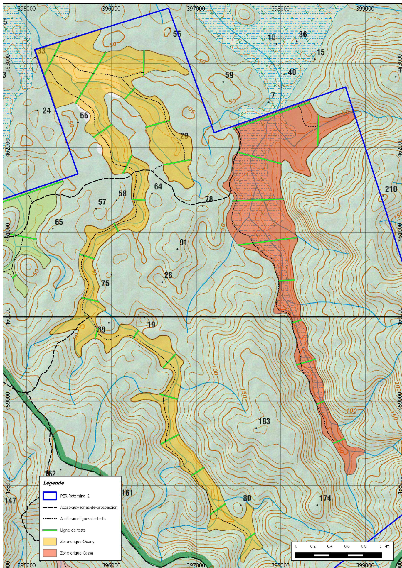
ANNEXE 4d : Plan de projet SANDS RESSOURCES - DOTM Puits de reconnaissance sur les zones n°4 (crique Ouany) et n°5 (crique Cassa) PER n°33-2019 d'après la carte IGN au 1/22 500° en UTM22, RGFG95
