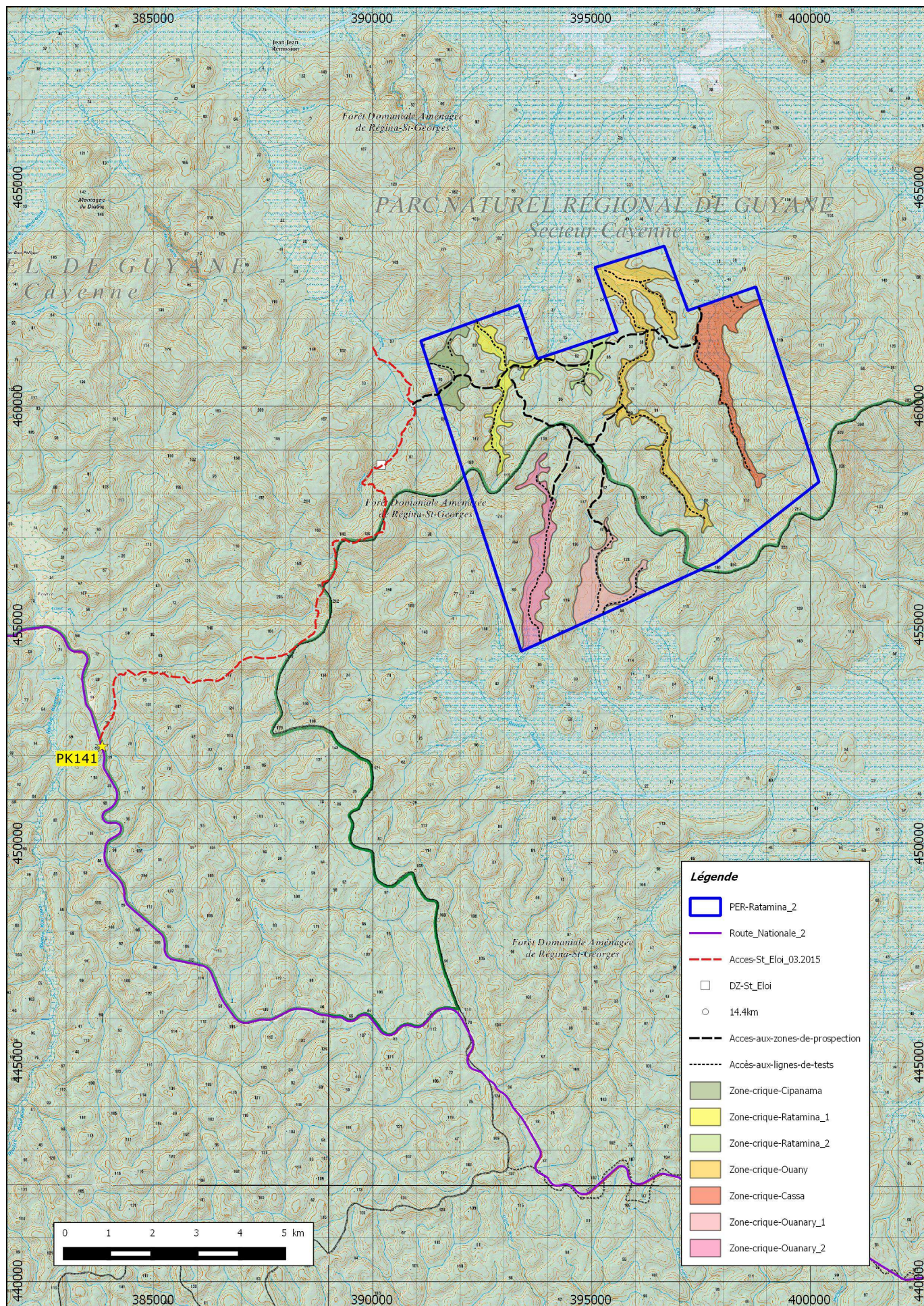
ANNEXE 4a : Accès au projet SANDS RESSOURCES - DOTM Puits de reconnaissance sur le PER n°13-2019 d'après la carte IGN au 1/50 000° en UTM22, RGFG95
