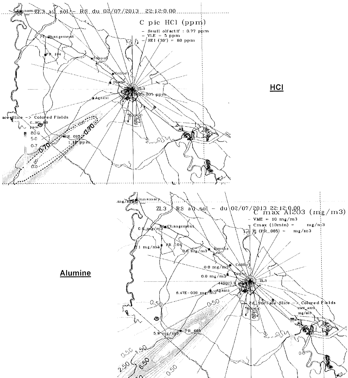
Figure 4 : Cartes de localisation des retombées au sol des produits de combustion suite au vol A212
