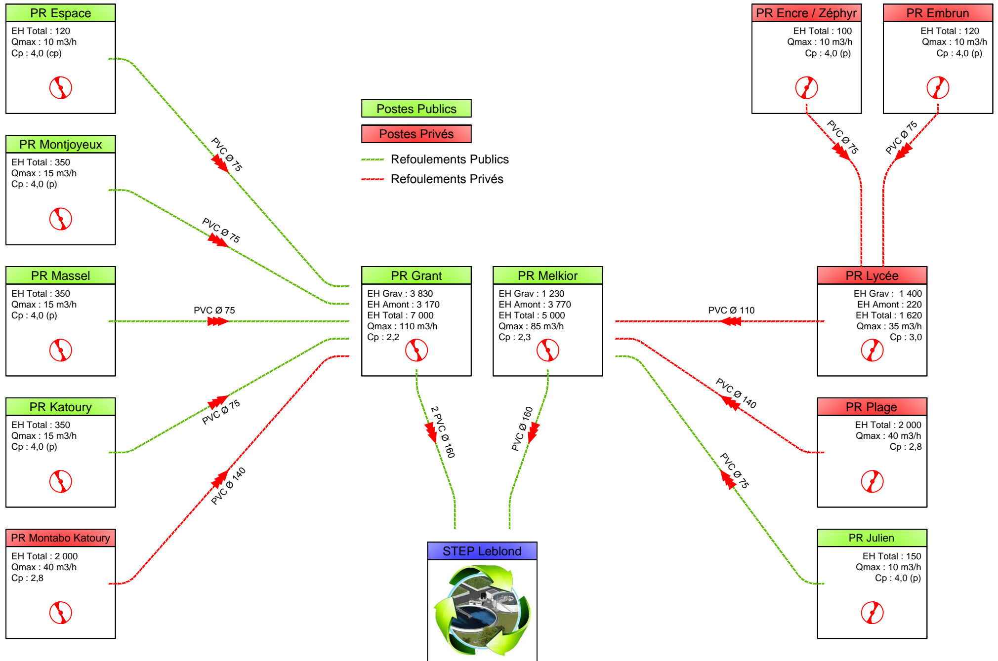
Assainissement des cités périphériques de Cayenne - Bassin Versant Montabo Nord Synoptique des postes de refoulement des eaux usées - Mai 2016
